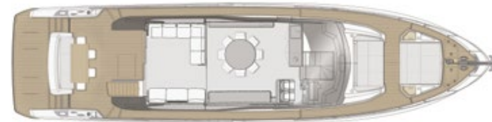
Hard Top version 硬顶版本
